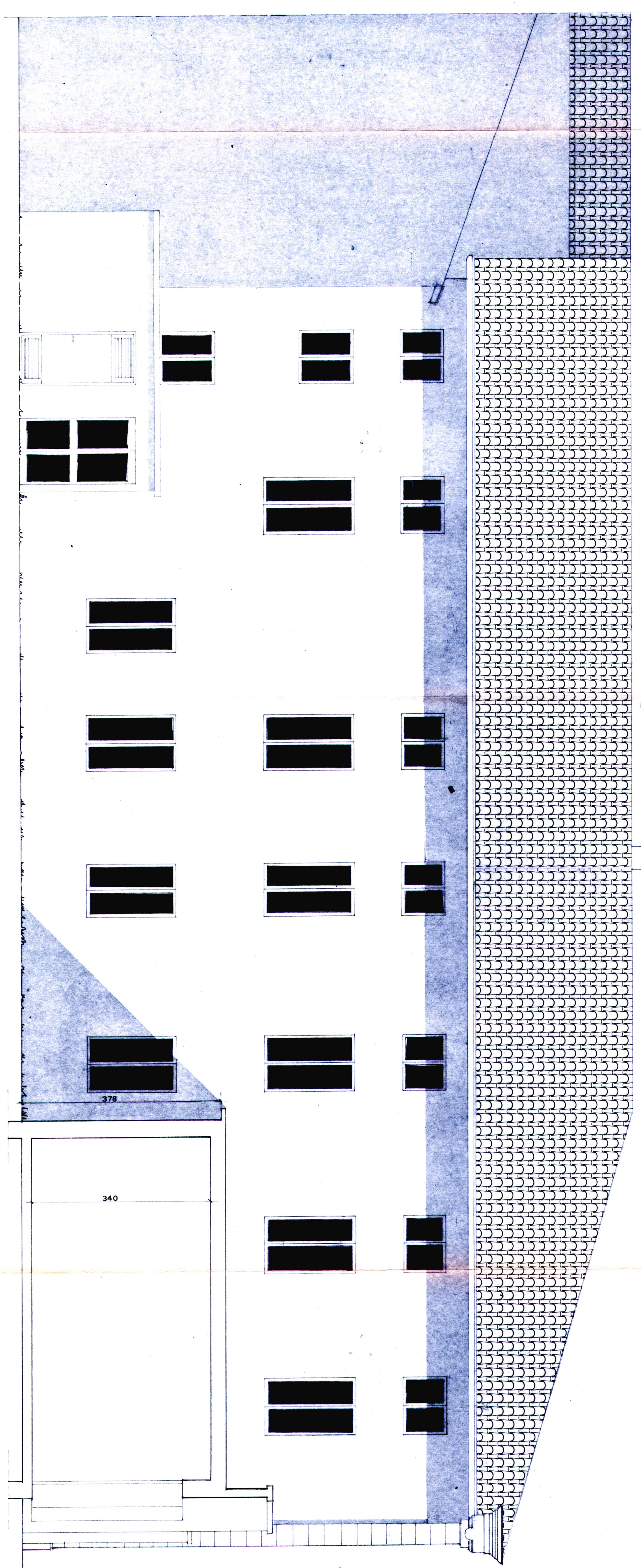
PROSPETTO SUL CORTILE CON SEZIONE B-B - 1:50
